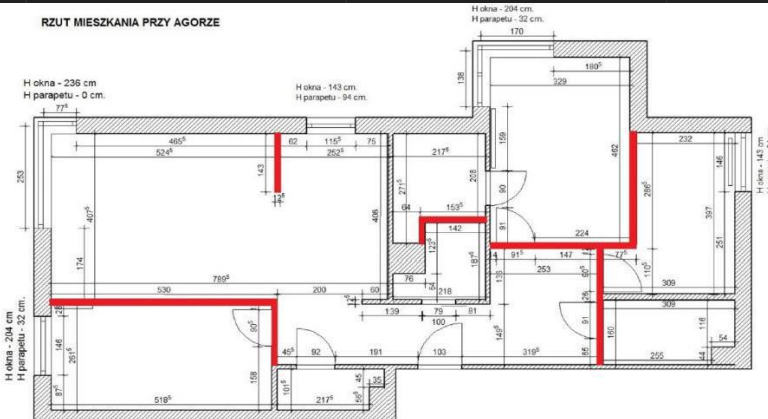
WYSOKOŚĆ POMIESZCZEN - 260 cm. WYSOKOŚĆ DRZWI - 208.9cm
